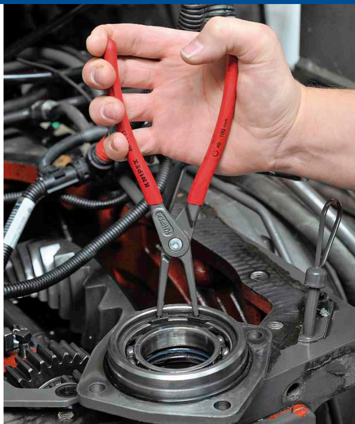
Прецизионные щипцы для стопорных колец для внутренних стопорных колец в отверстиях
